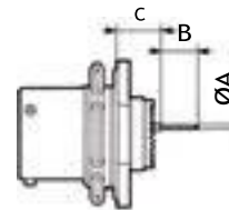
Type 7 Jam nut receptacle
