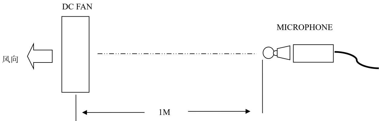
7-1.噪音测试方法示意图（Schematic diagram of noise test method）：
