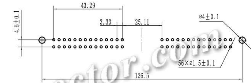
PCB板孔示意图 PCB BOARD HOLE DIAGRAM
