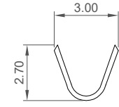
Sec:A-A
