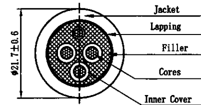
SEC A-A
