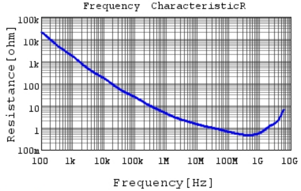
GCM155L81H471KA37 R DCOV, 25degC
