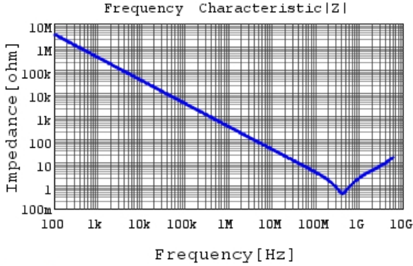
GCM155L81H471KA37 |Z| DCOV, 25degC
