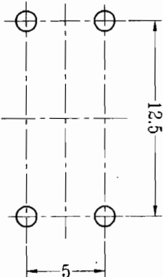
P.C.B LAYOUT
