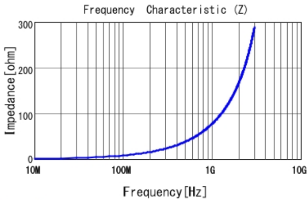
LQW15AN12NG0Z |Z|
