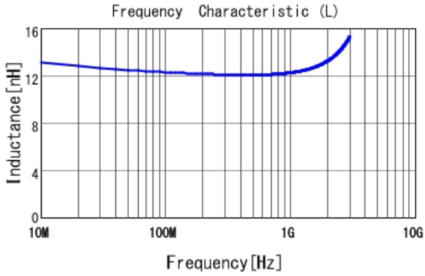
LQW15AN12NG0Z L
