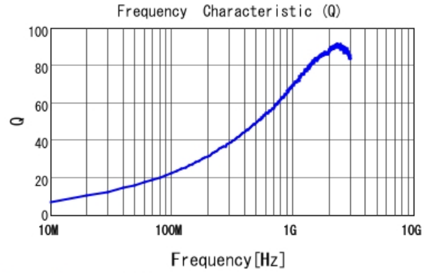
LQW15AN12NG0Z Q
