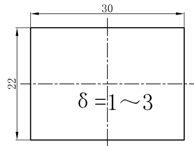
安装面板尺寸 PANEL CUT-OUT
