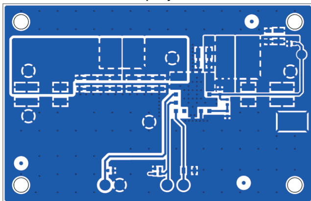
Layer 3 (Single)
