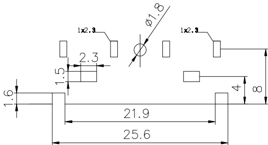
PCB开孔尺寸
