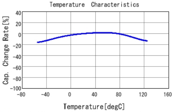
■ GRT033C71A104KE01 C-Temp. capchange, DCO. 0V, ACO. 2Vrm
