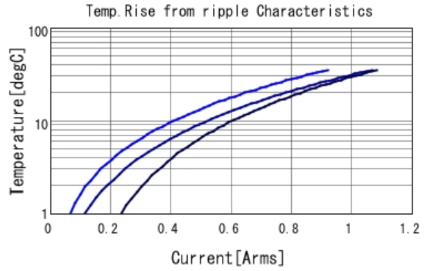
GRT033C71A104KE01 Temp. rise ■ 400kHz ■ 800kHz ■ 1MHz
