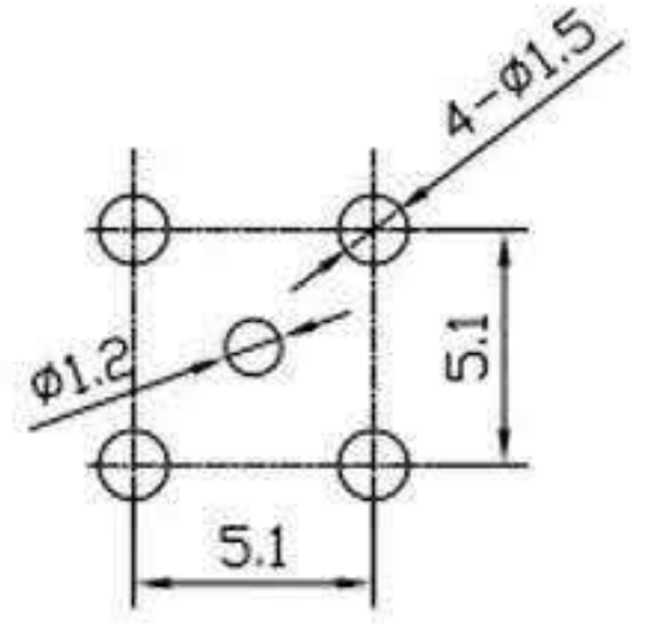
PCB参考图
