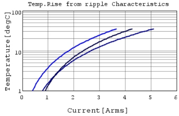
GRT21BC71H475KE13 Temp.rise — 100kHz —
