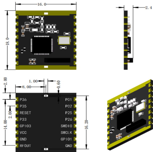
图 2. 模块尺寸图
