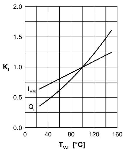
Fig. 4 Typ. dynamic parameters Q_r , I_{RM} versus T_{VJ}
