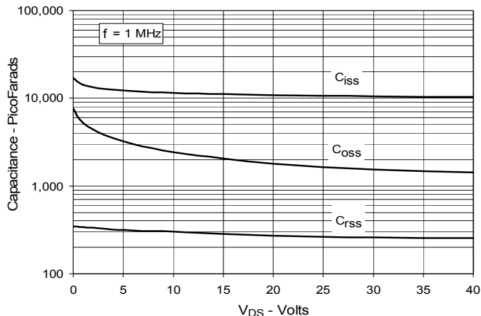
Fig. 11. Capacitance
