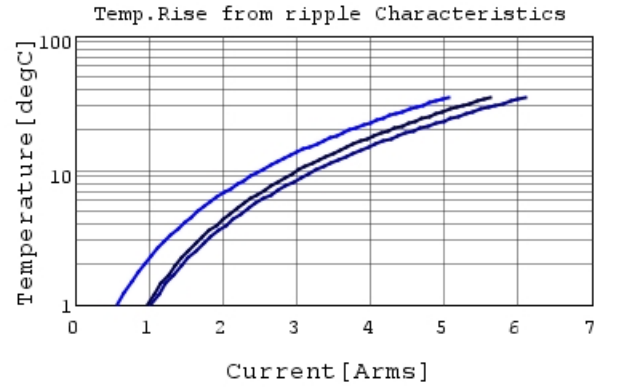
GRM219R61C226ME15 Temp.rise — 80kHz —
