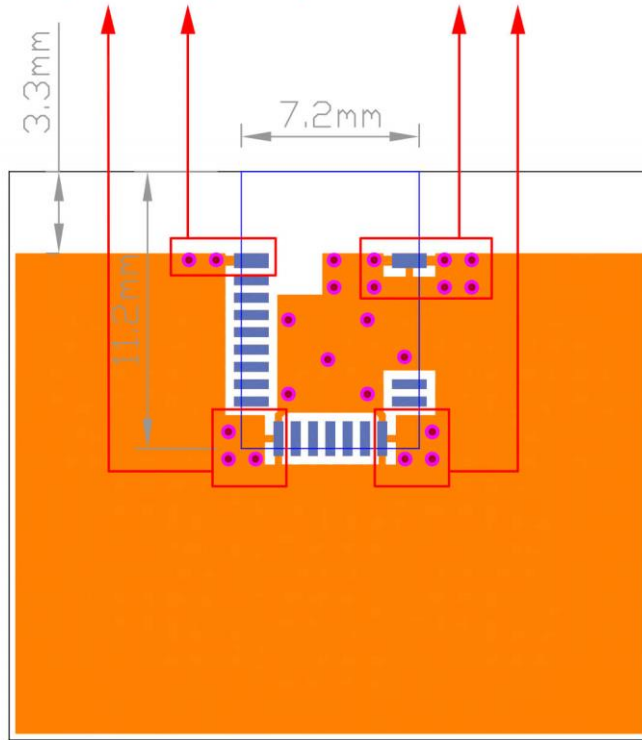
Top layer
