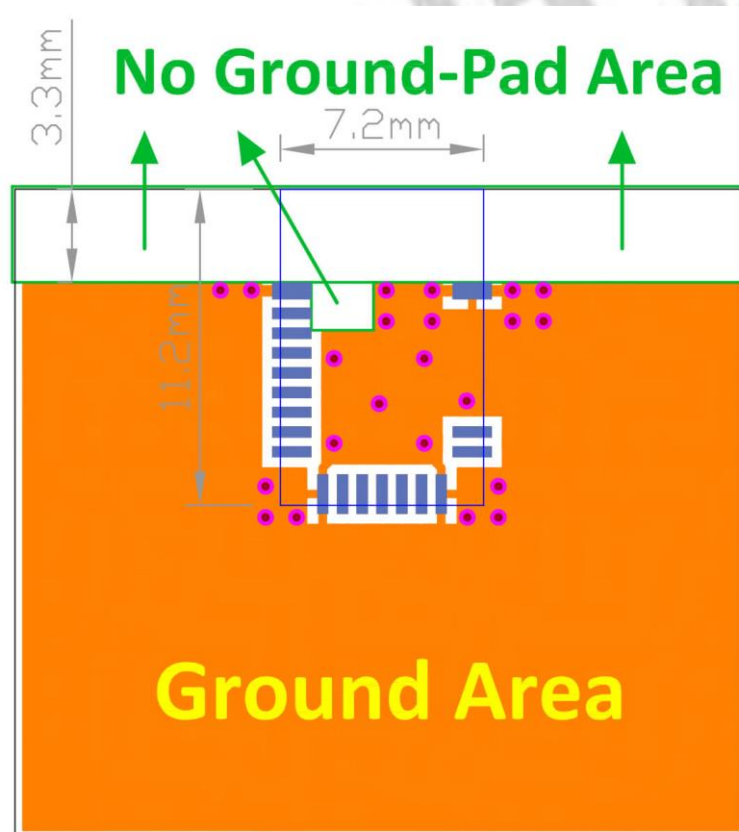
Top layer
