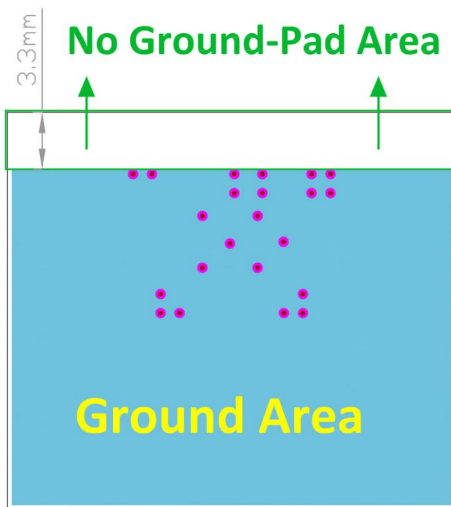
Bottom layer
