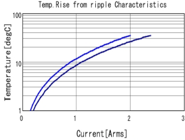
GRM155R70J105KA12 Temp. rise ■ 500kHz ■ 1MHz
