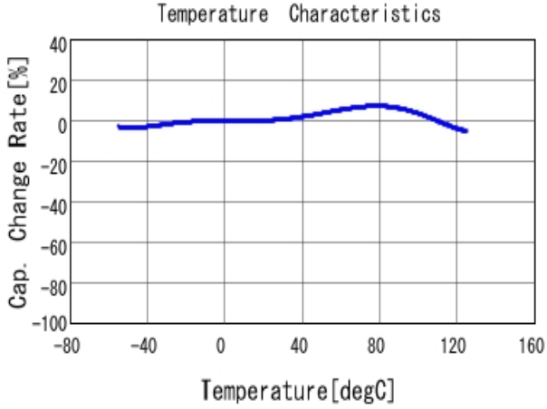
■ GRM155R70J105KA12 C-Temp. capchange, DCO. 0V, ACO. 5Vrm
