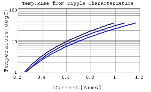
GRM1555C1E150JA01 Temp.rise — 500MHz
