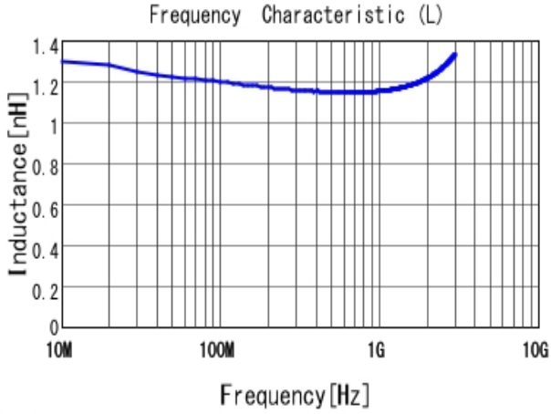
■ LQG15HZ1N2C02 L
