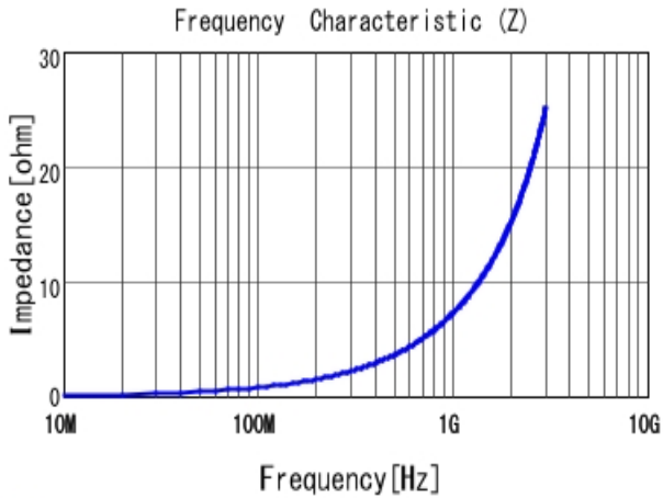
■ LQG15HZ1N2C02 |Z|
