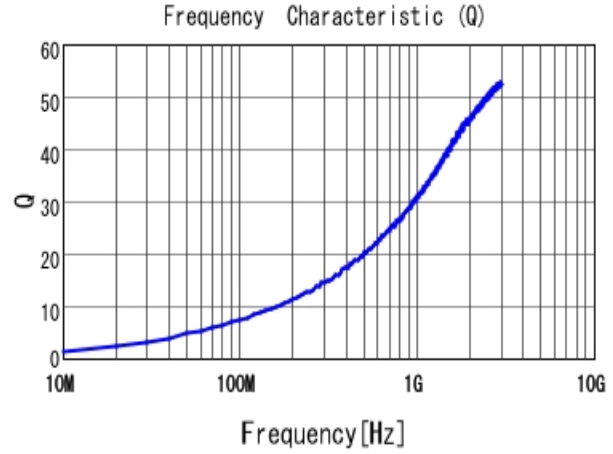
■ LQG15HZ1N2C02 Q
