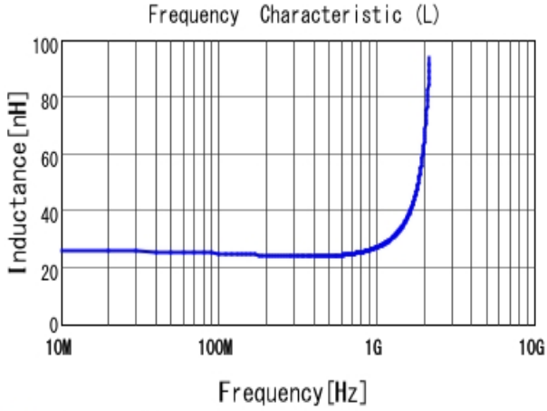
■ LQP03TG24NH02 L
