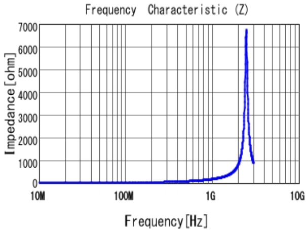
■ LQP03TG24NH02 |Z|
