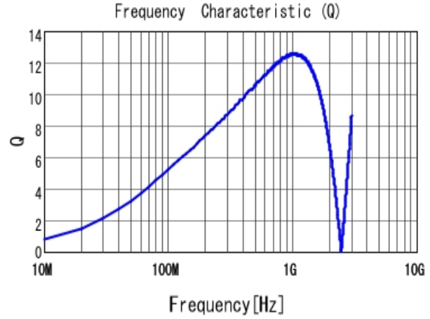
■ LQP03TG24NH02 Q
