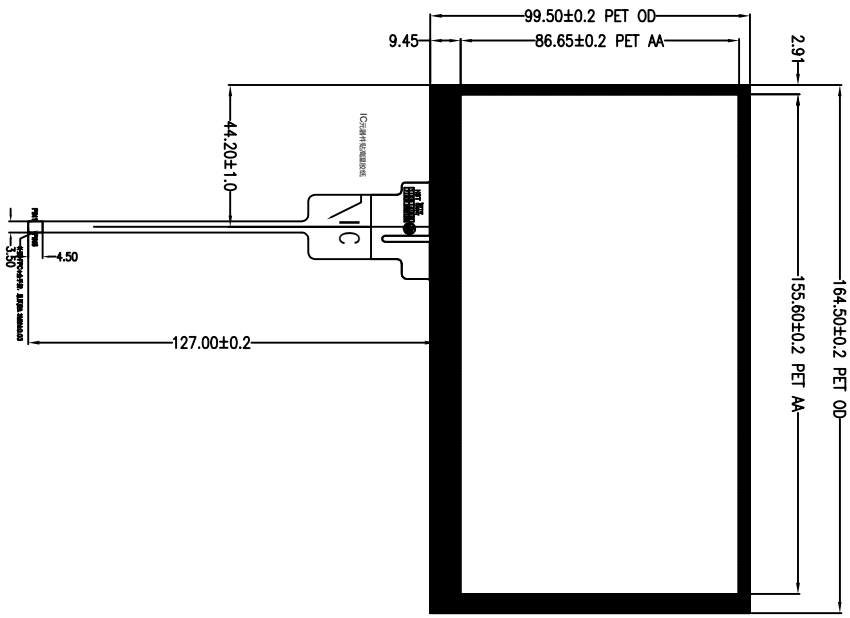
正视图
