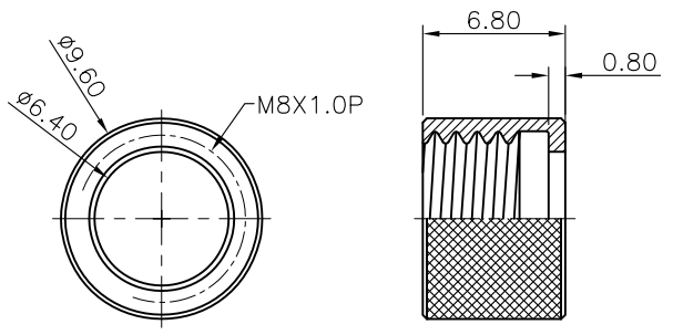
NUT
