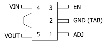
SOT-89-5L
