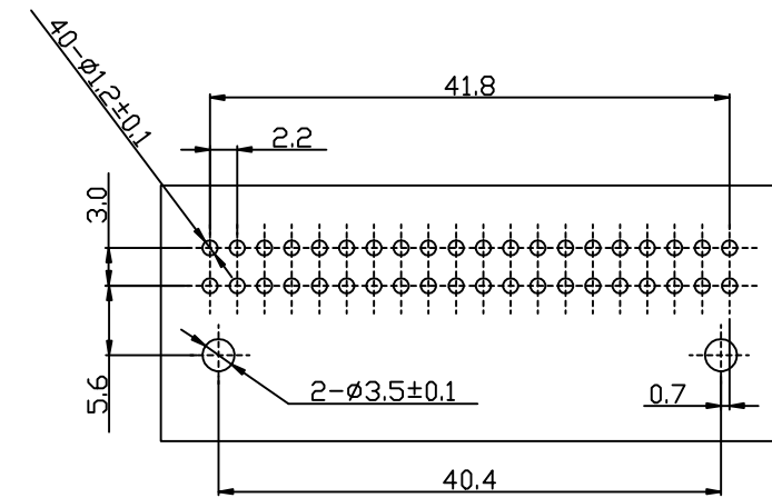
PCB 板孔示意图
