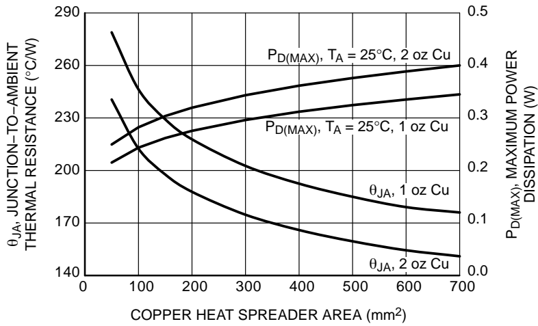
Figure 45. θ JA vs. Copper Area (uDFN4)
