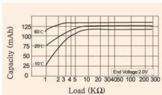
电阻容量曲线
