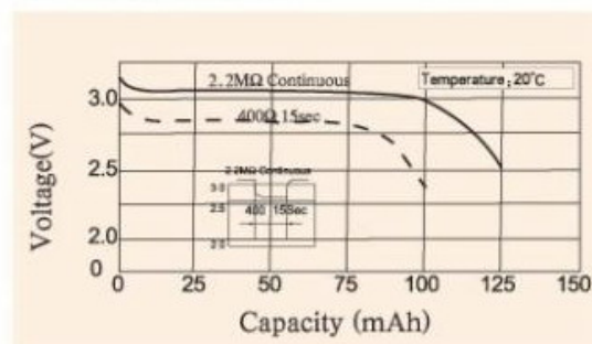
脉冲放电曲线
