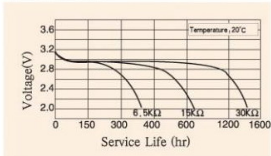
电阻容量曲线
