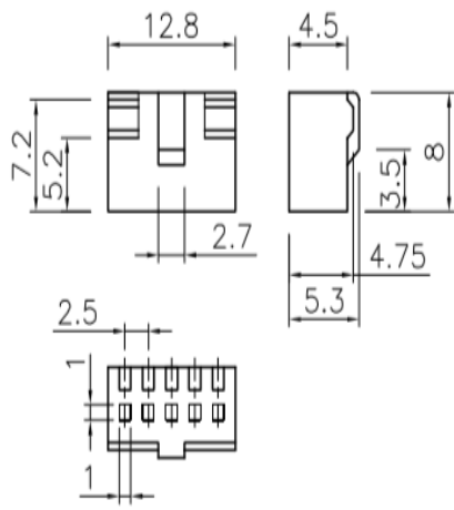
DET. A
