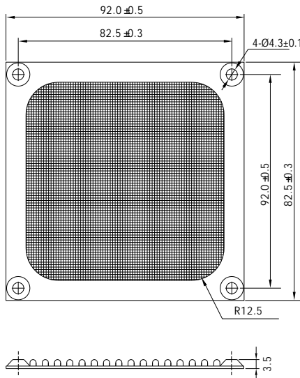
MF Ø9 For 90mm Fan
