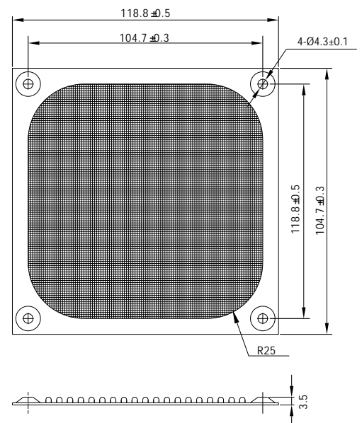
MF 12 For 120mm Fan
