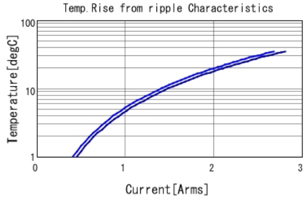
GRM033R60G225ME47 Temp. rise ■ 500kHz ■ 1MHz
