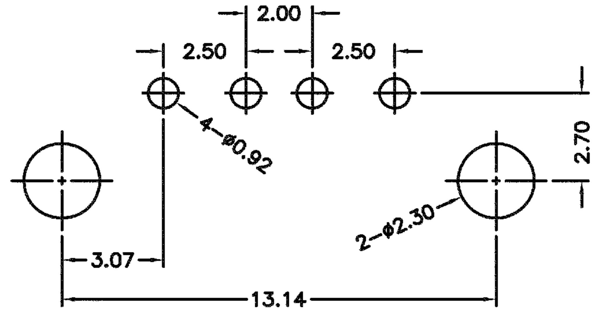
P.C.B. LAYOUT
