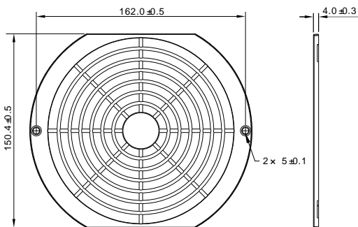
PG 17 For 172mm Fan
