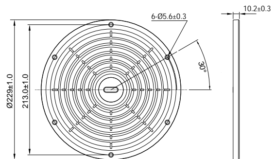
PG 20 For 200mm Fan
