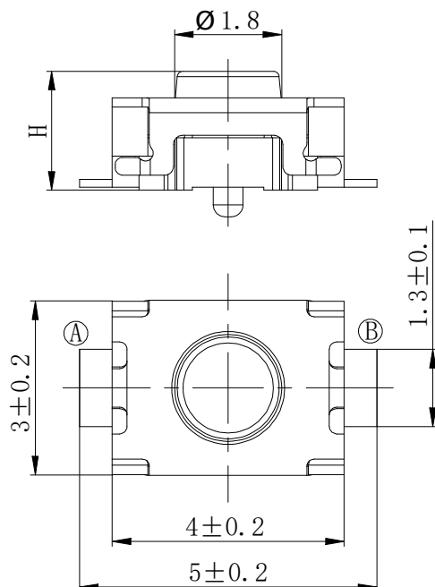
焊接尺寸图
