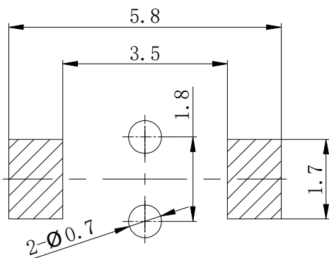
焊接尺寸图
