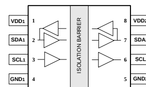
CMT8101 NB SOIC-8/ WB SOW-8
