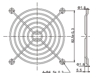
PFG-90 For 90mm Fan
