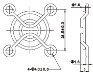
PFG-30 For 30mm Fan
