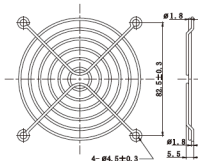
PGF-60 For 60mm Fan
