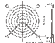
PFG-90 For 90mm Fan
