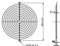
PFG-170 For 150mm Fan
