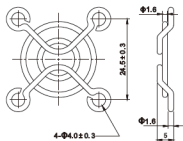
PFG-30 For 30mm Fan
