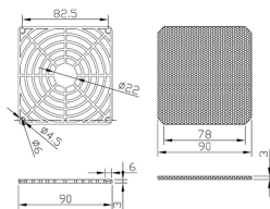
PFGF-90 For 90mm Fan
