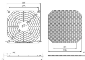
PFGF-120 For 120mm Fan
