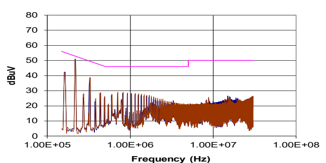
NMV0505TSAC (Average)
