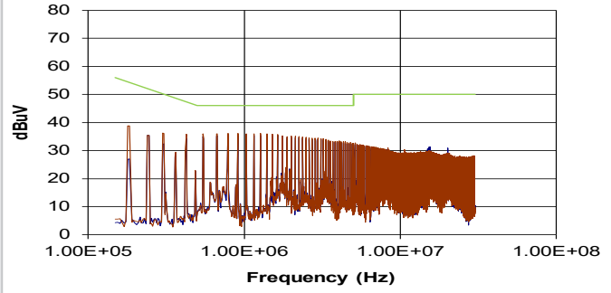
NMV0512TSC (Average)
