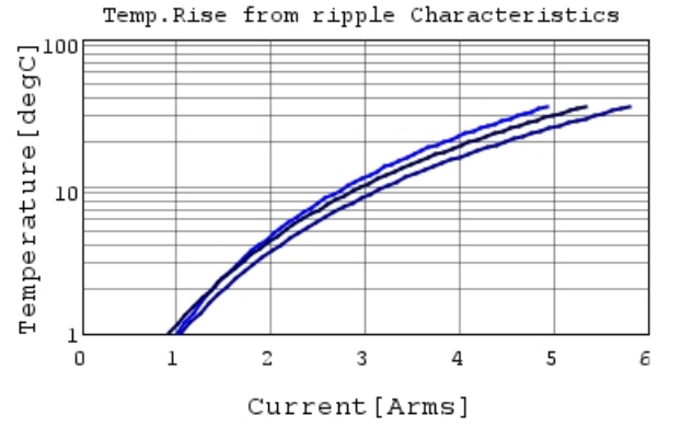
GRM31CR61C106KA88 Temp.rise — 100kHz
