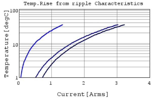
GRT155R61C474KE01 Temp.rise — 200kHz —
