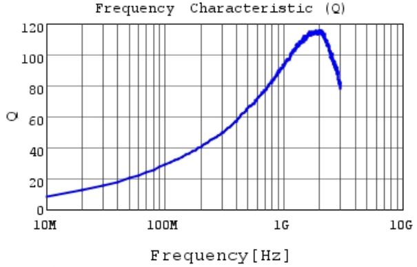
LQW18AN13NG00 Q
