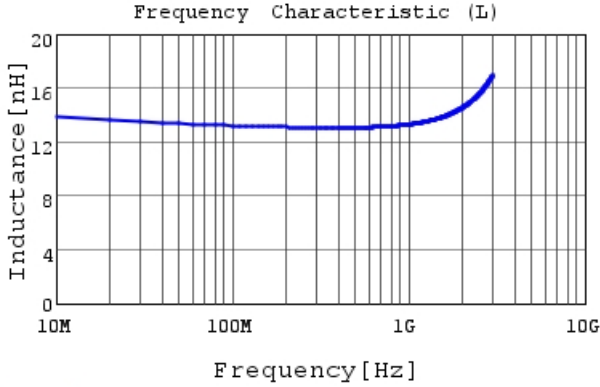
LQW18AN13NG00 L
