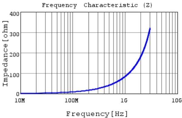
LQW18AN13NG00 |Z|
