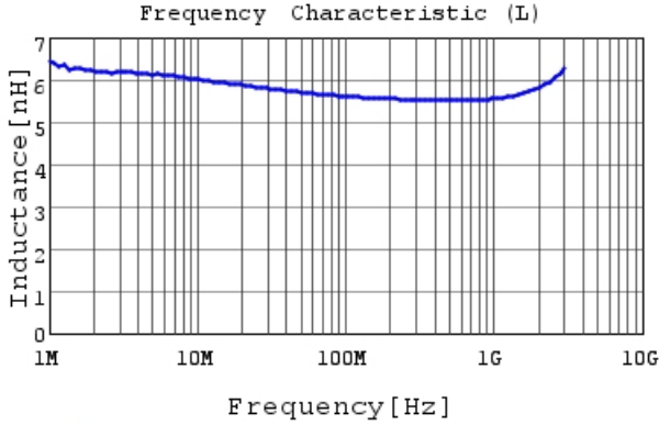
LQW15AN5N6B80 L
