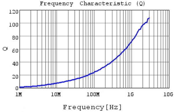
LQW15AN5N6B80 Q
