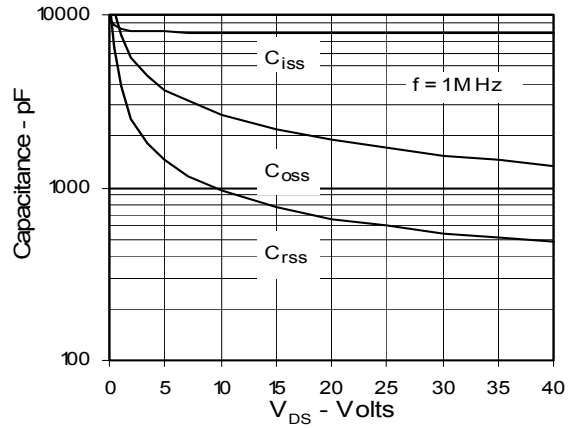
Fig. 10. Capacitance
