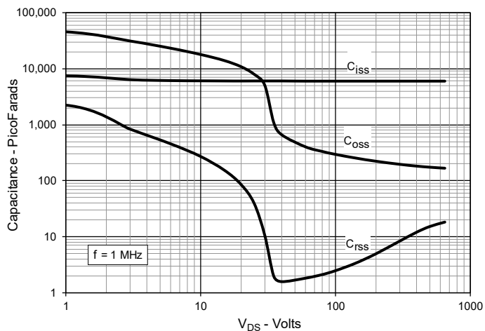
Fig. 12. Capacitance
