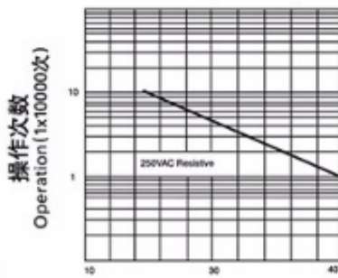
电气寿命曲线 LIFE Expectancy
