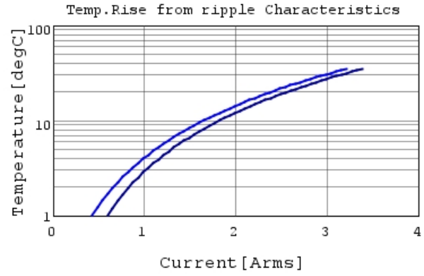
GRT155R61A225KE01 Temp.rise — 500kHz —
